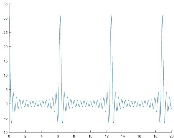
Figure: Fourierserien med N = 15 för ett impulståg med period 2\pi .
