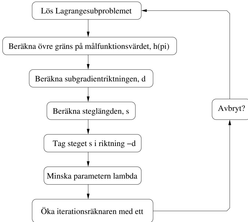
Figure 2: Beräkningsschema.
