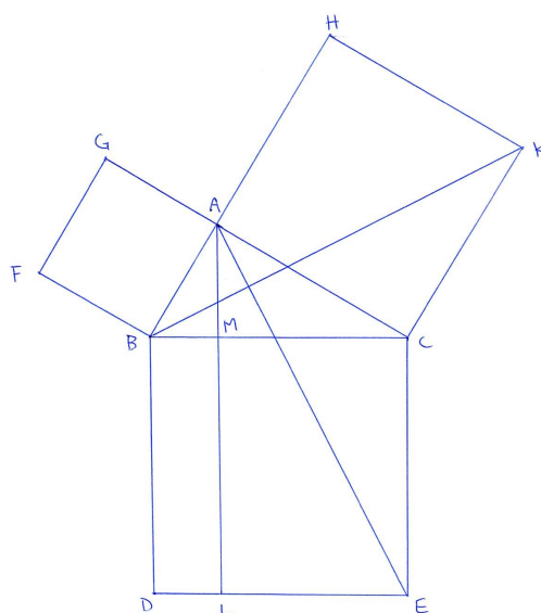
Figur 8: Om sträckorna mellan punkt B och K respektive punkt A och E dras och samma resonemang som innan förs, så påvisas att arean av kvadraten CKHA är lika stor som arean på rektangeln MCEL.
