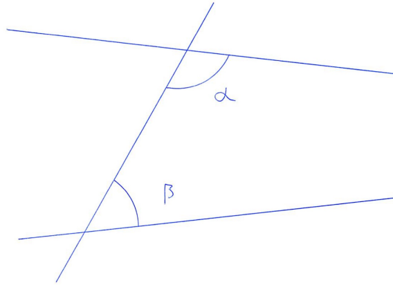
Figur 1: Parallellpostulatet säger att vinkelsumman av vinkeln \alpha och vinkeln \beta , som bildas när transversalen skär de två linjerna, ska vara mindre än två rätta vinklar (2R), det vill säga 180^\circ , för att linjerna vid förlängning ska korsa varandra. Ekvivalent så innebär detta att det går att dra en och endast en linje genom en punkt utanför en given linje så att de båda linjerna blir parallella.
