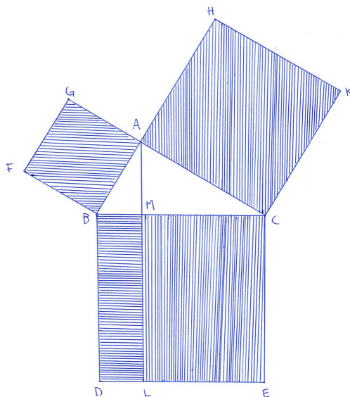
Figur 9: Åskådning av kvadraterna på sidan BA och AC, vars sammanlagda area svarar mot den summerade arean av de rektanglar som tillsammans utgör kvadraten på sidan BC.
