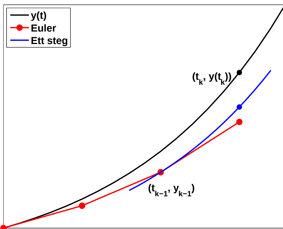
Lokalt och globalt fel
