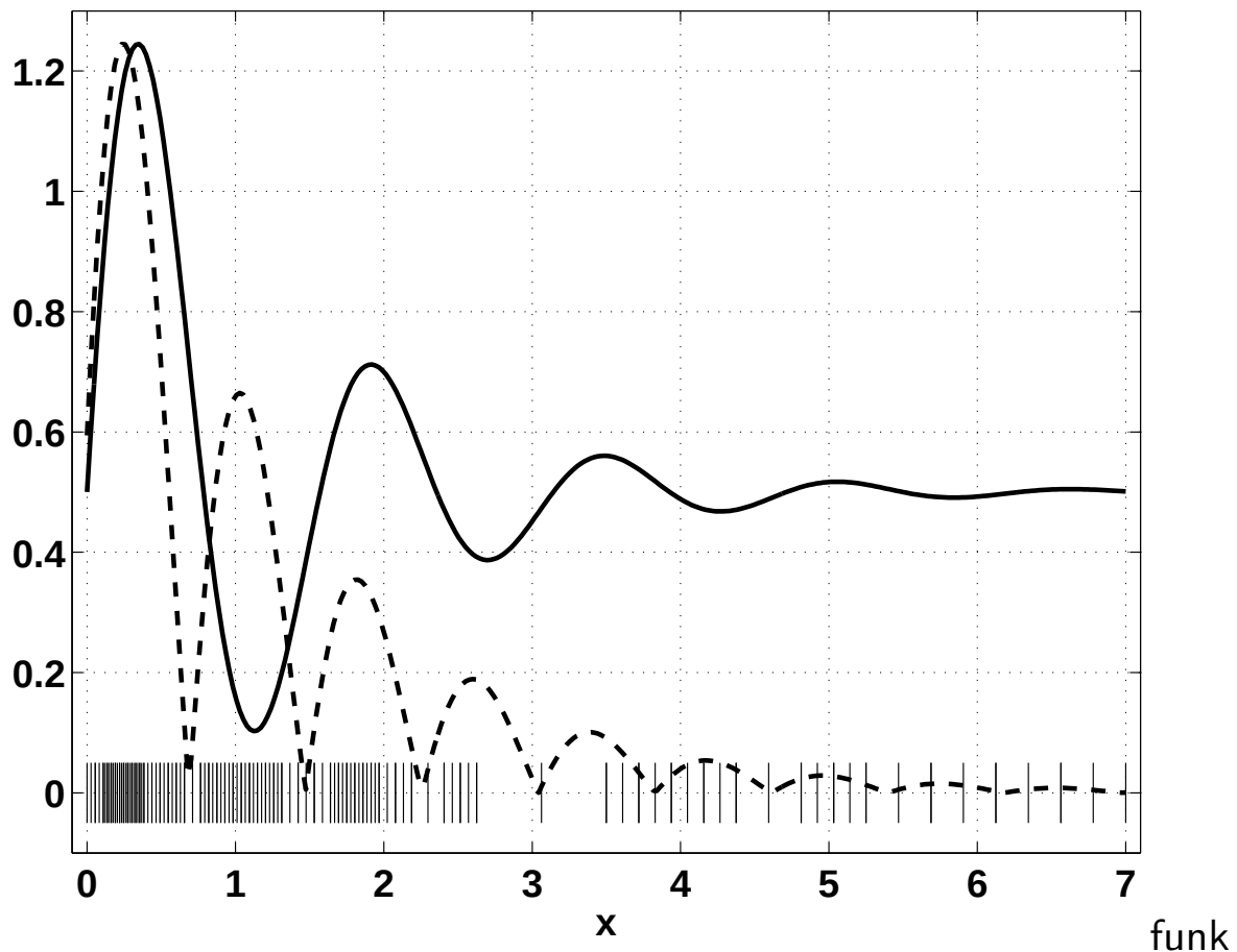
En rekursiv trapetsmetod. Skalande |f''(x)| --, f(x) -.
