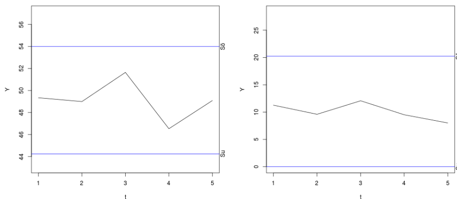
(a) Medelvärdesdiagrammet
