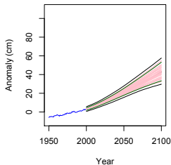
RCP 2.6
