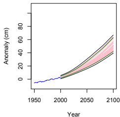
RCP 6.0
