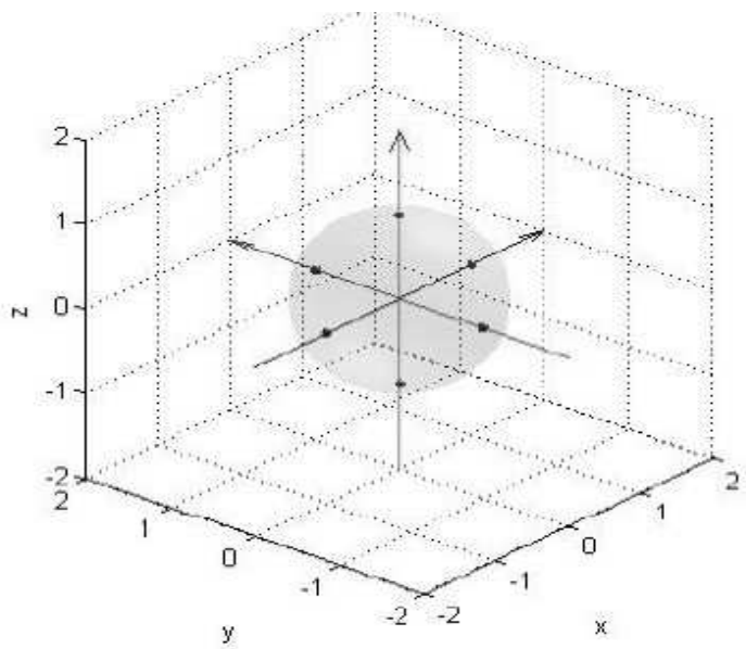
Figur 1: Sex punkter på enhetssfären i 3D, transformerade till koordinataxlarna
