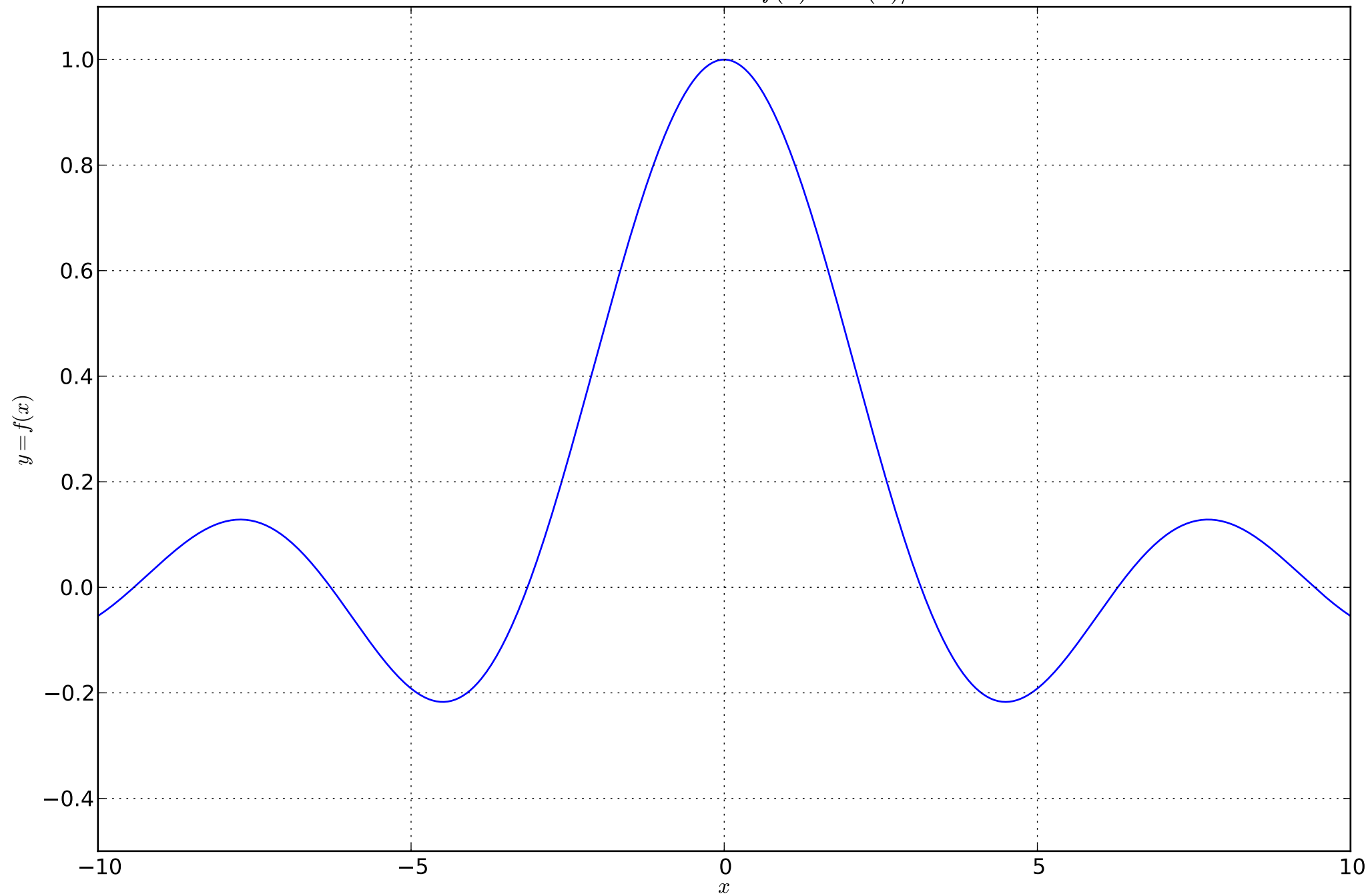
Plot av funktionen f(x) = \sin(x)/x
