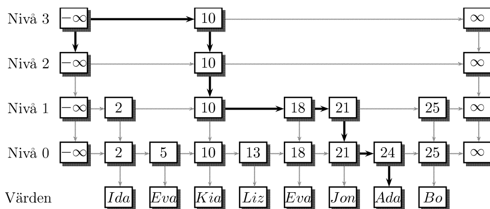
Figure 1: Exempel på skiplista med nycklarna 2,5,10,13,18,21,24,25
