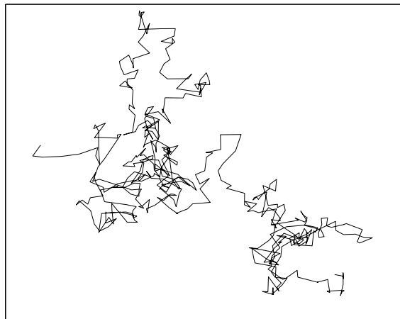
Figur 1.3: Brownsk rörelse
