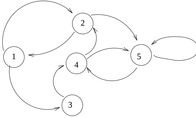
Figur 3.1: Övergångsgraf
