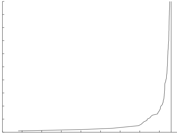
Figur 6.5: Exploderande födelseprocess.
