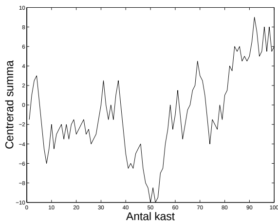
Figur 1.4: Centerad följd av tärningskast
