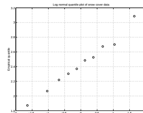
Figur 3: En kvantilplot av snödatamängden i övning 5. Teoretisk modell är den lognormala.
