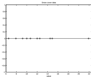
Figur 1: En illustration av snödatamängden i övning 5.
