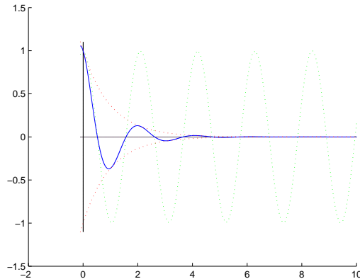
FIGUR 1. u(t) = e^{-t} \cos(3t) tillsammans med \pm e^{-t} och \cos(3t) .
